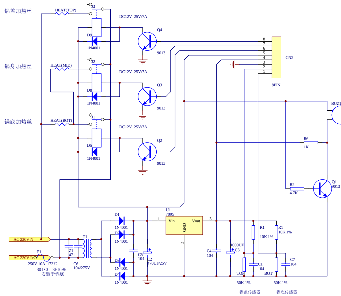
30FC4电源板
