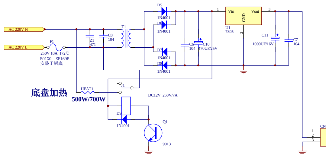
30YD1 40YD1 50YD1 30YC1 40YC1 50YC1电源板
